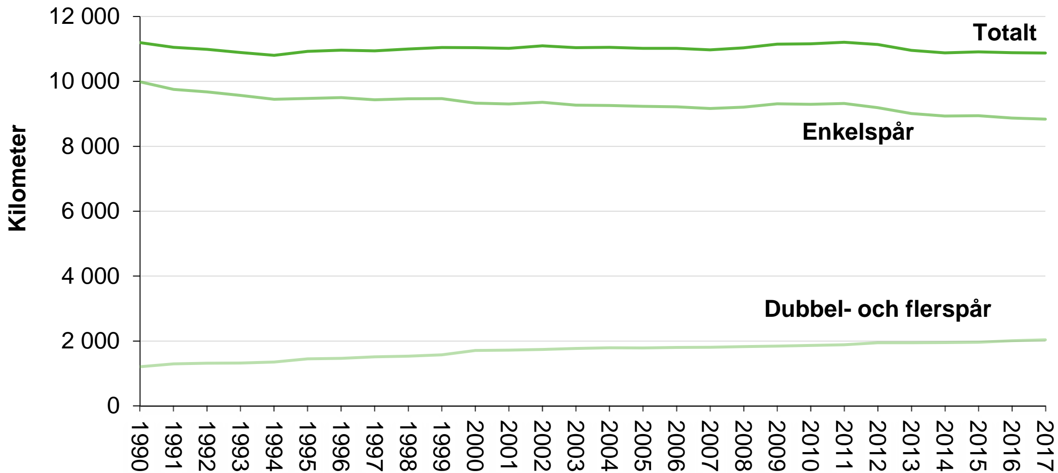
Figur 1.1. Trafikerad banlängd för järnvägar fördelad på antal spår 1990–2017.
