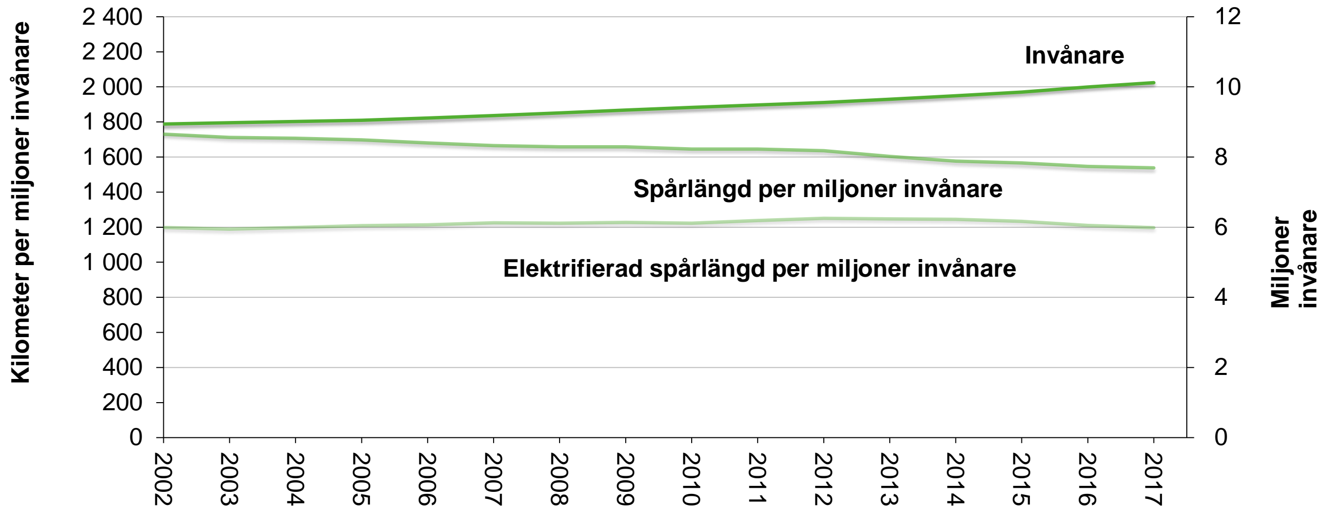
Figur 1.2. Trafikerad spårlängd för järnvägar per miljoner invånare och antal invånare 2002–2017. Källa för invånare: SCB:s statistikdatabas avläst 2018-06-04.
