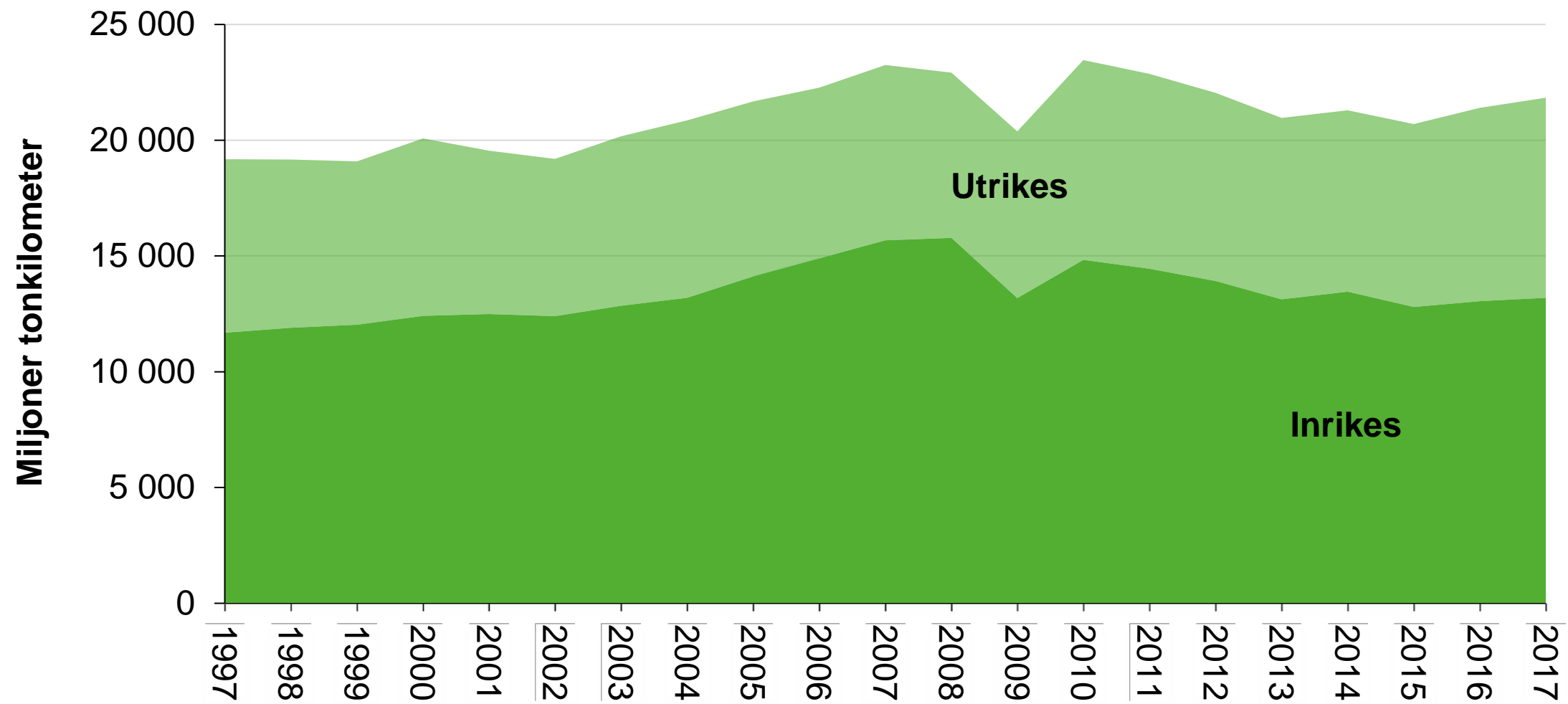
Figur 4.4. Godstransportarbete med järnväg, fördelat på inrikes och utrikes 1997–2017.
