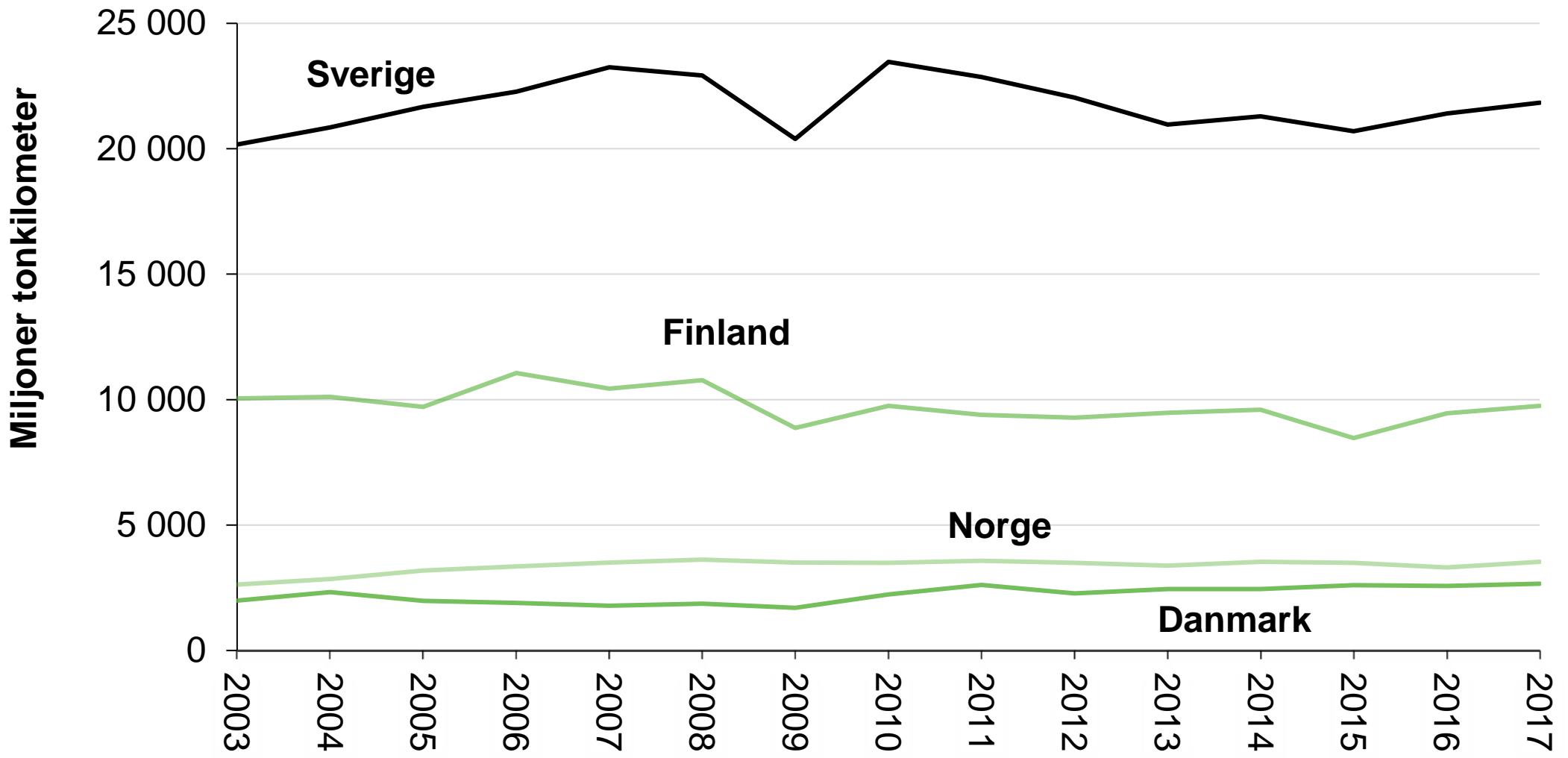
Figur 6.1. Godstransportarbete i nordisk jämförelse 2003–2017. Anm: Danmarks, Finlands och Norges uppgifter är preliminära för år 2017.
