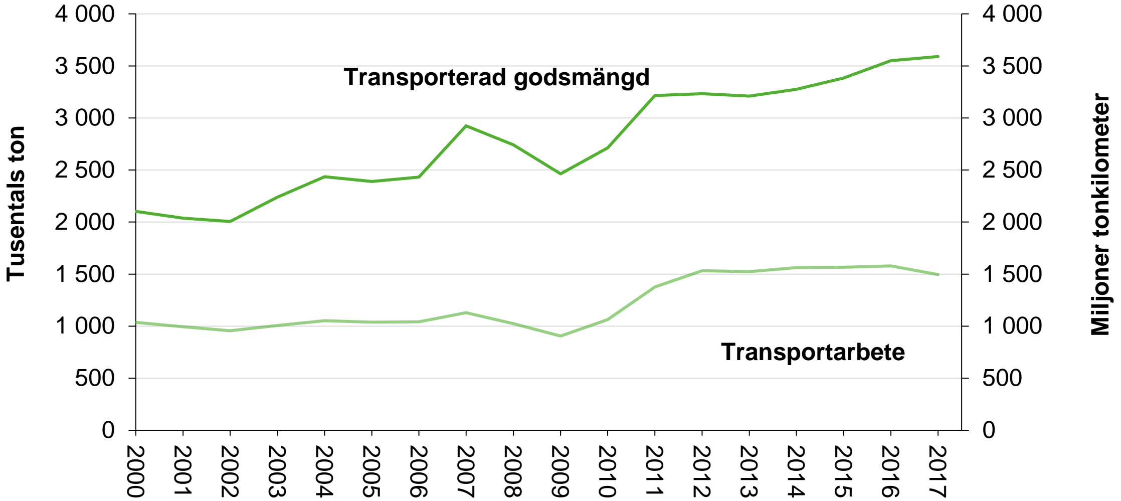
Figur 4.2. Transportarbete för farligt gods i tonkilometer och transporterad mängd farligt gods i ton på järnväg 2000–2017.
